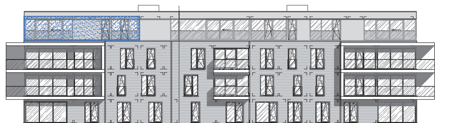
ACHTERGEVEL
